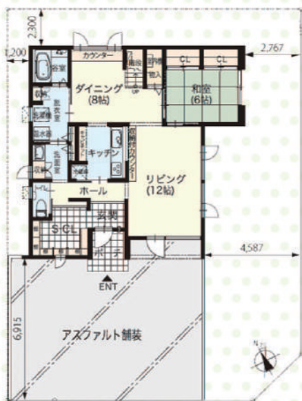
1階平面図・配置図
